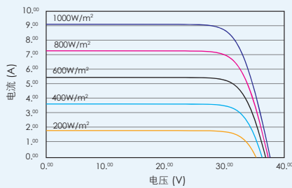
组件的I-V曲线 (260W)
